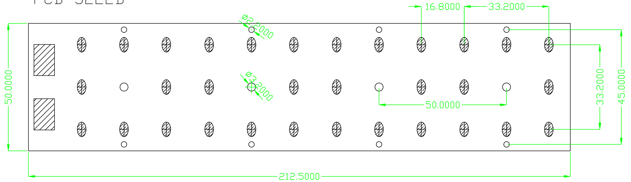
PCB 32LED
